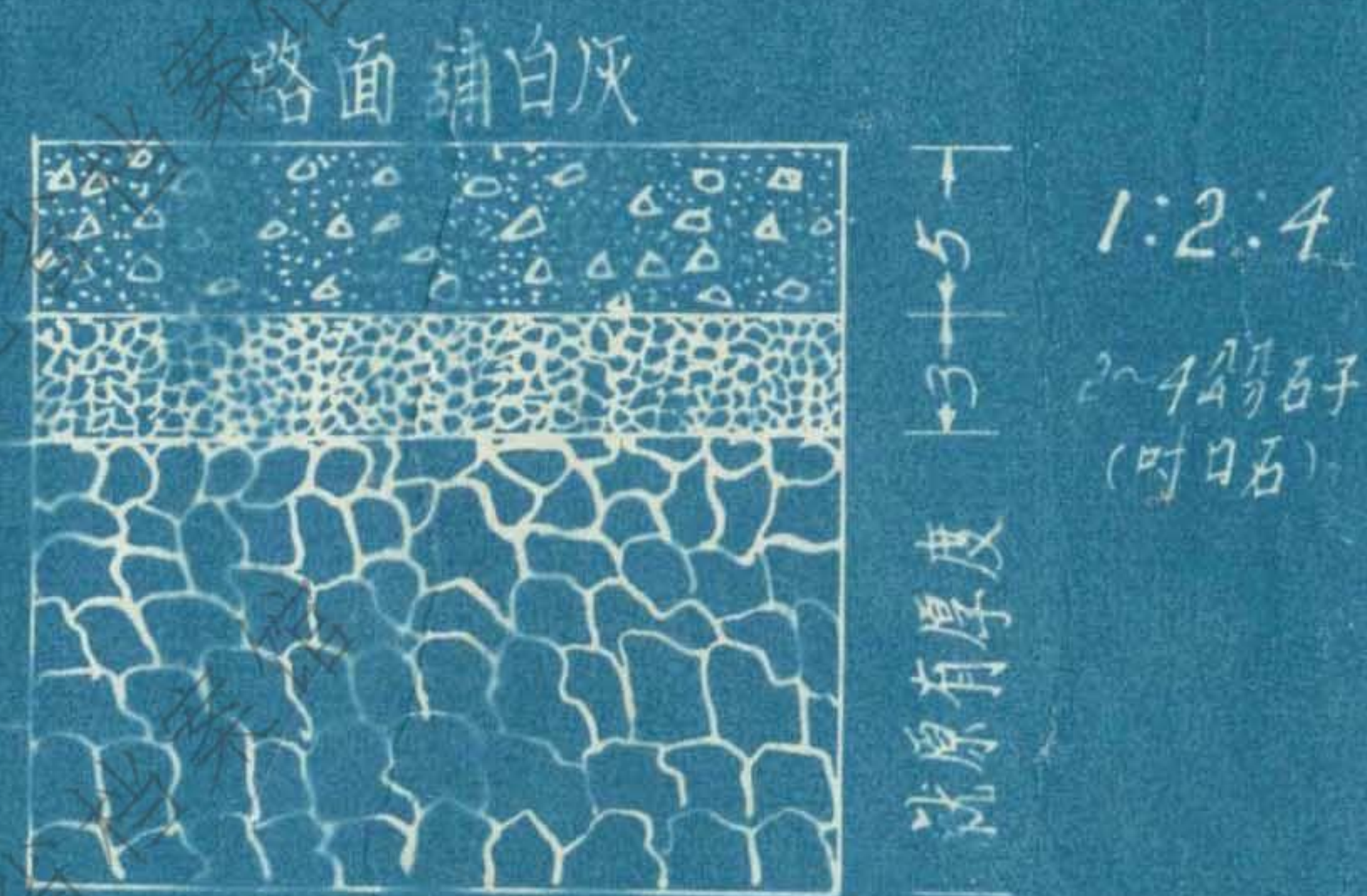
圖一 路面詳圖 比例 1:50
