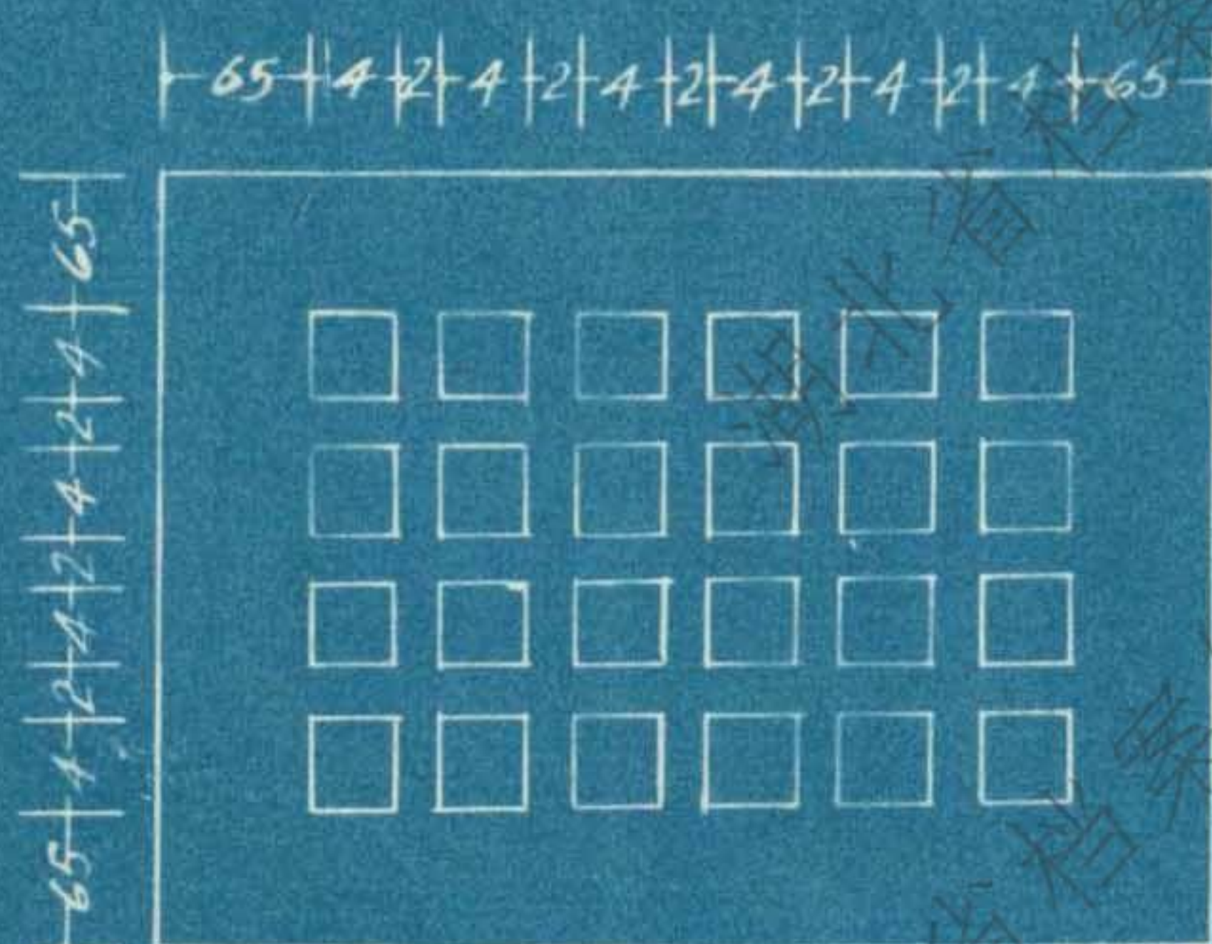
木蓋板 圖三 比例 1:10
